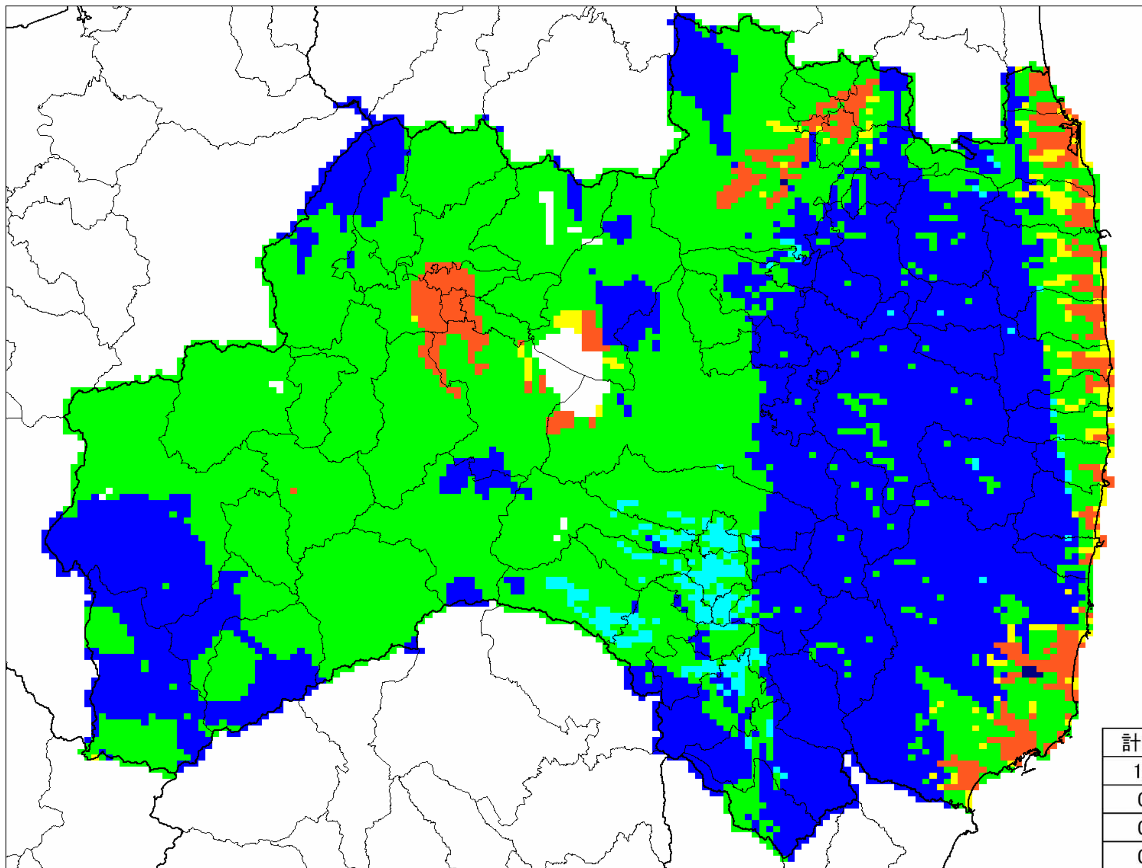
図 表層地盤のゆれやすさ (福島県)
